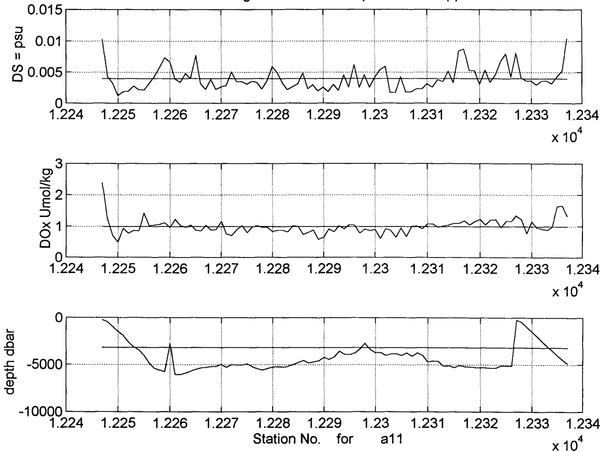
Figures 9a, 9b and 9c: CTD DQE
